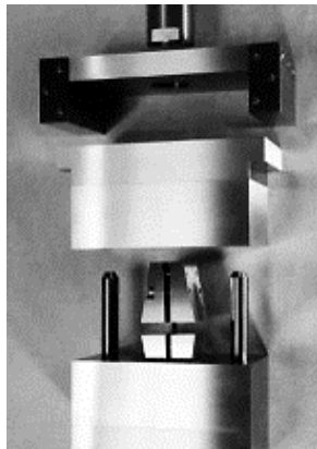
圧縮試験
