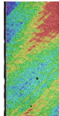
ひずみ分布例 (CFRP)
