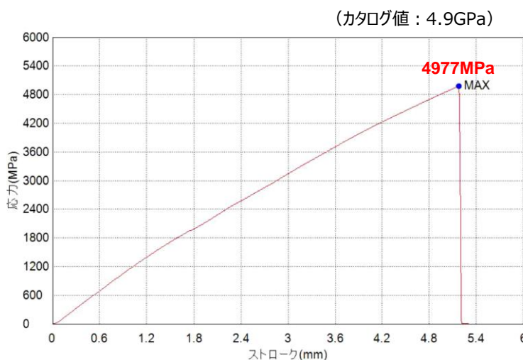
応力・ストローク線図
